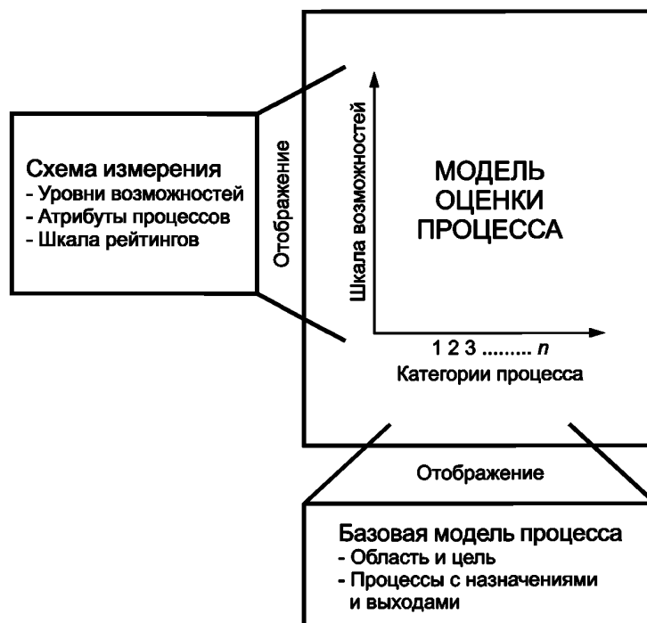
Рисунок 5 — Взаимосвязи модели процесса оценки
