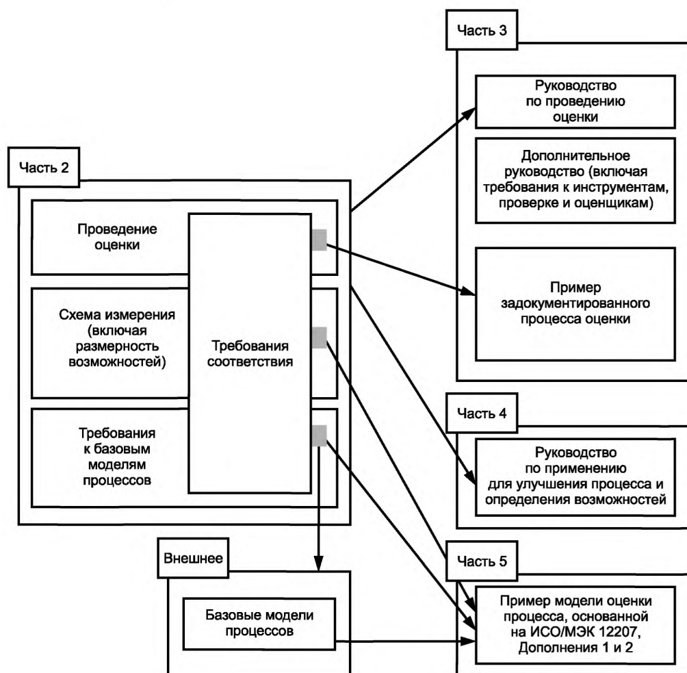
Рисунок 3 — Обзор взаимосвязей между элементами серии стандартов ИСО/МЭК 15504
