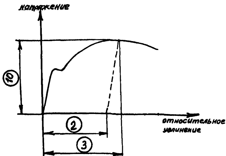
Рисунок 1 - Схема определения относительного удлинения \delta_p, \delta_b Примечание - Пояснения к номерам, заключенным в круг, см. в таблице 1
