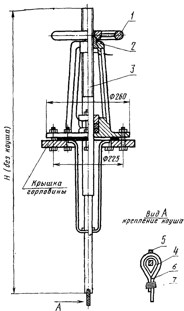
1—маховик; 2—стойка; 3—шпиндель; 4—коуш; 5—подвеска; 6—канат; 7—оплетка
