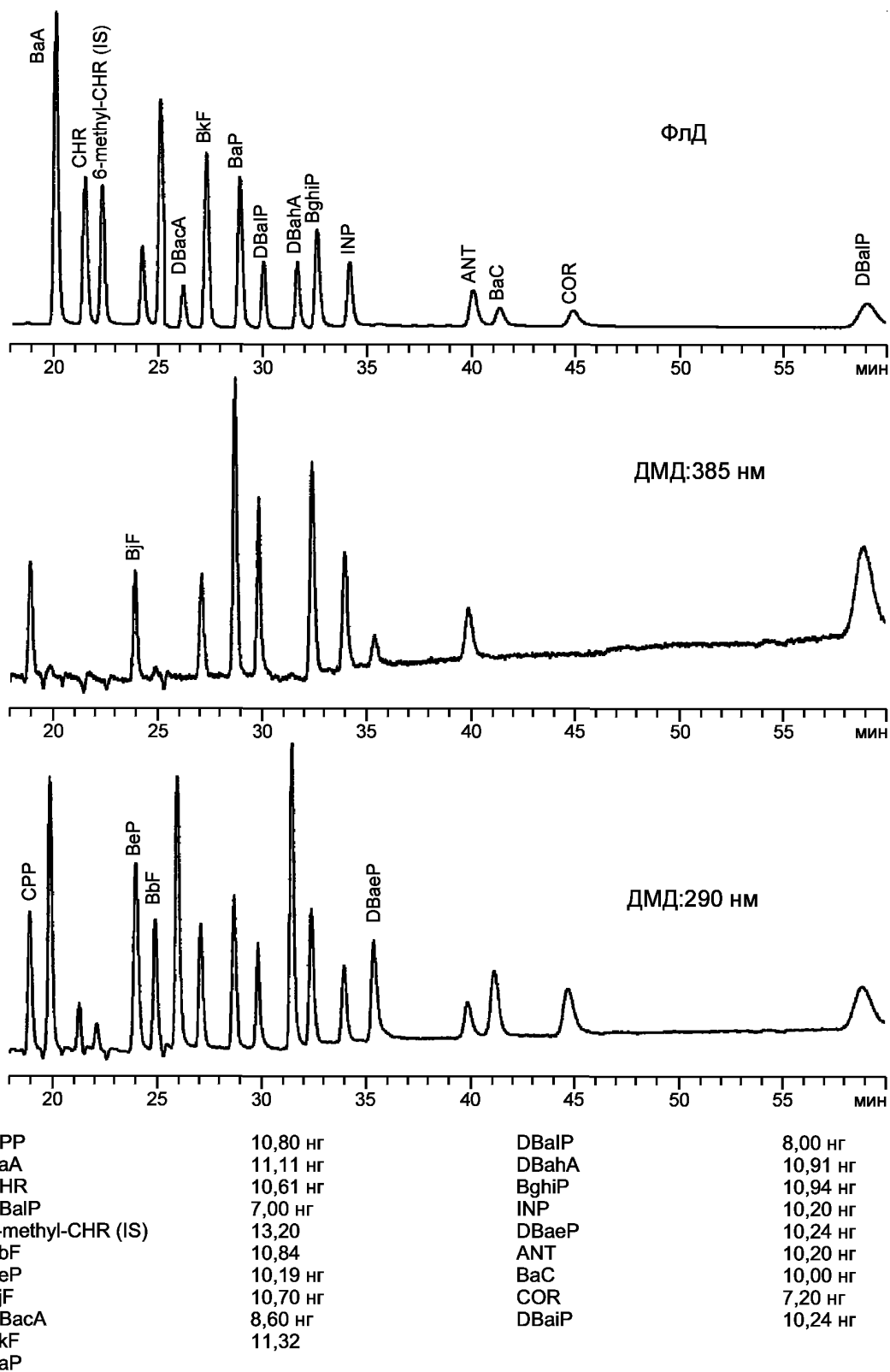
Рисунок В.1 — Хроматограмма градуировочной смеси ПАУ
