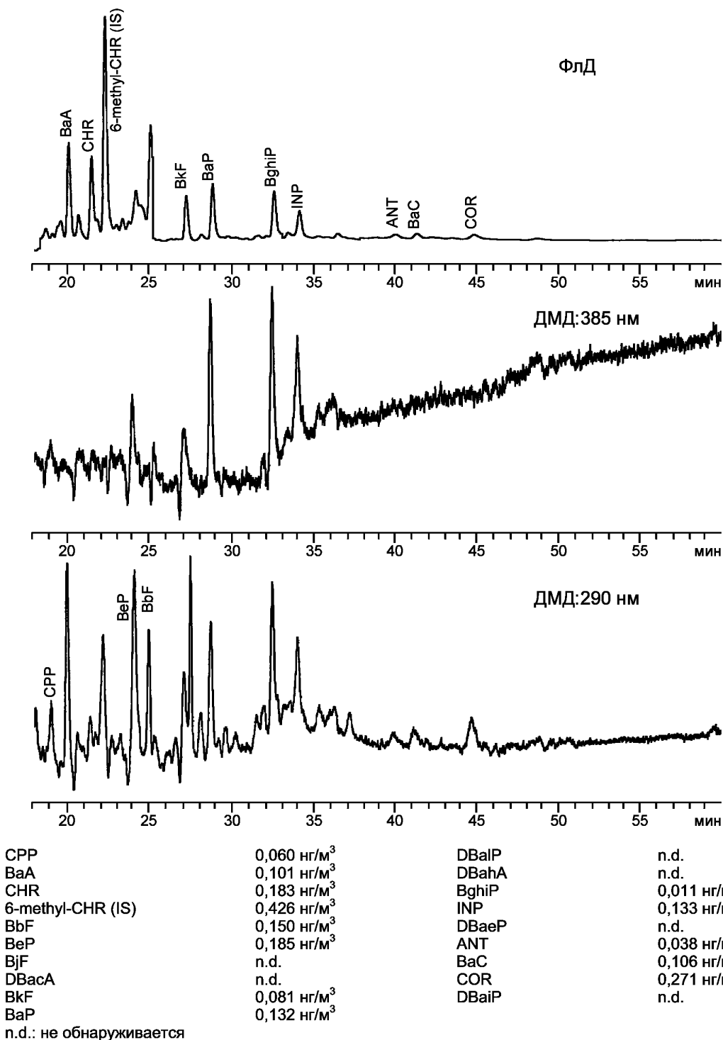
Рисунок В.2 — Хроматограмма пробы воздуха
