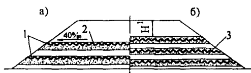
Рисунок 8.5 – Применение ГМ при возведении земляного полотна из грунтов повышенной влажности
