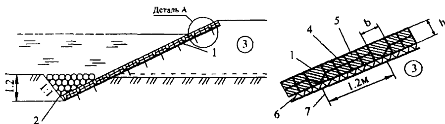
1 — георешетка; 2 — каменная призма; 3 — земляное полотно; 4 — синтетический трос; 5 — заполнитель георешетки; 6 — фильтр из геотекстильного материала; 7 — анкер; h и b — высота и ширина ячейки георешетки
