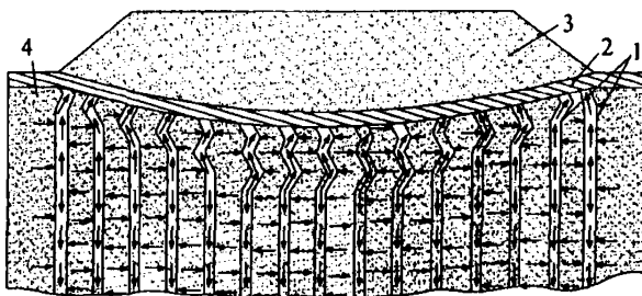
1 – ленточные дрены; 2 – песчаный слой; 3 – насыпь; 4 – слабое основание
