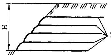
Рисунок 11.5 – Применение ГМ для повышения общей устойчивости откосов
