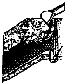
а – устройство фильтра из геотекстильного материала; б – укладка пространственной георешетки; в – заполнение ячеек георешетки
