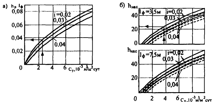
Рисунок 9.6 — Номограмма к расчету дренающего слоя (определение h_{\text{нас}} и C )
