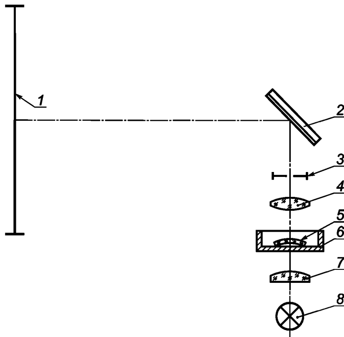
1 — экран для наблюдения со шкалой; 2 — зеркало; 3 — диафрагма; 4 — объектив; 5 — измеряемая контактная линза; 6 — опора контактной линзы (ювета); 7 — конденсор; 8 — источник света
