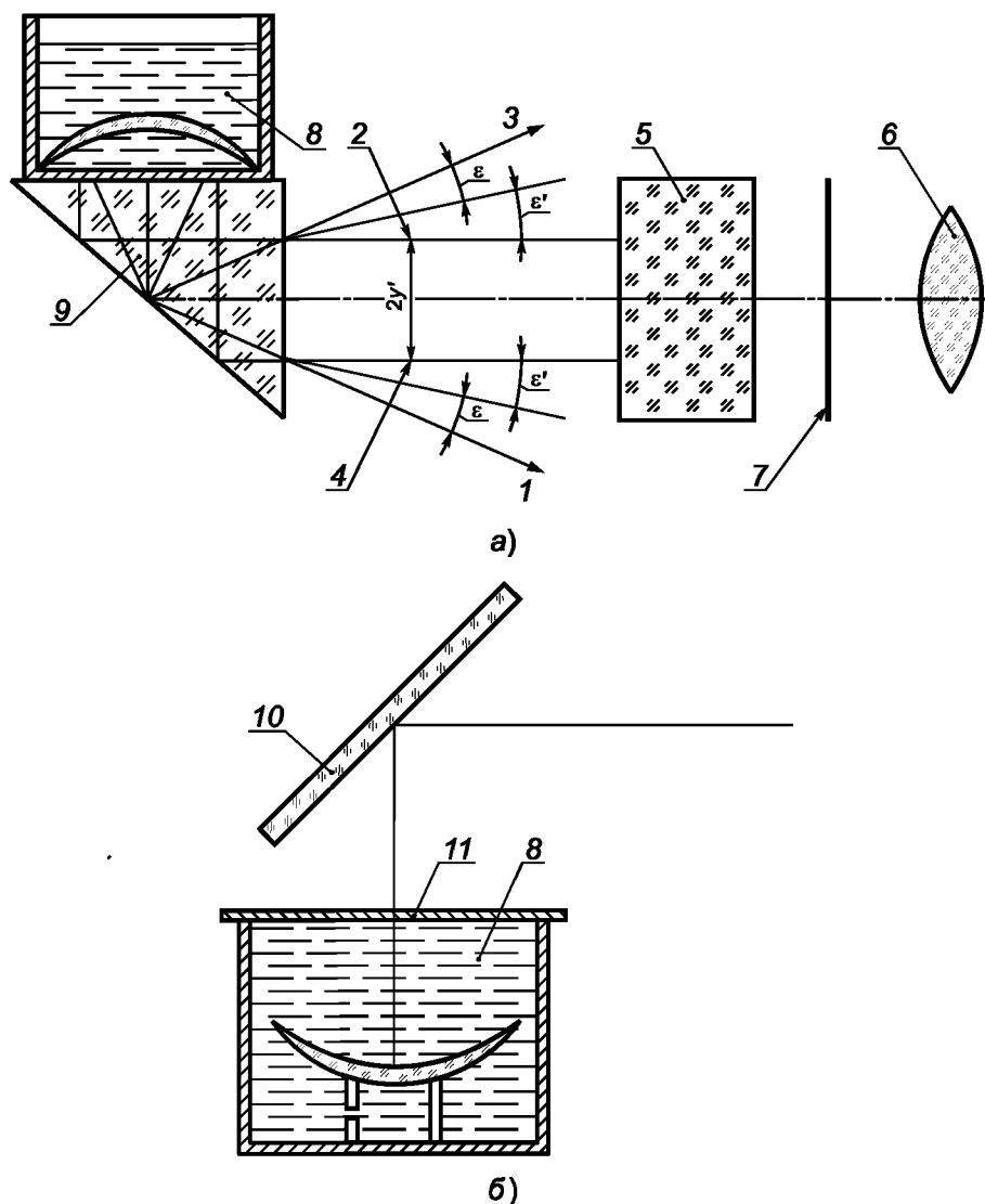
\varepsilon, \varepsilon' — углы падения; 2u' — расстояние между отраженными изображениями; 1 — мира 1; 2 — изображение мира 1; 3 — мира 2; 4 — изображение мира 2; 5 — система удвоения с объективом; 6 — окуляр; 7 — плоскость изображения объектива совпадает с плоскостью изображения окуляра; 8 — солевой раствор; 9 — призма; 10 — фронтальная поверхность посеребренного зеркала; 11 — прозрачная съемная крышка
