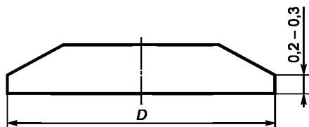
Рисунок 10 — Калибровочный диск
