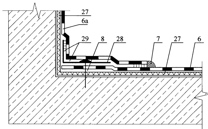
Узел 1.2 - 2
