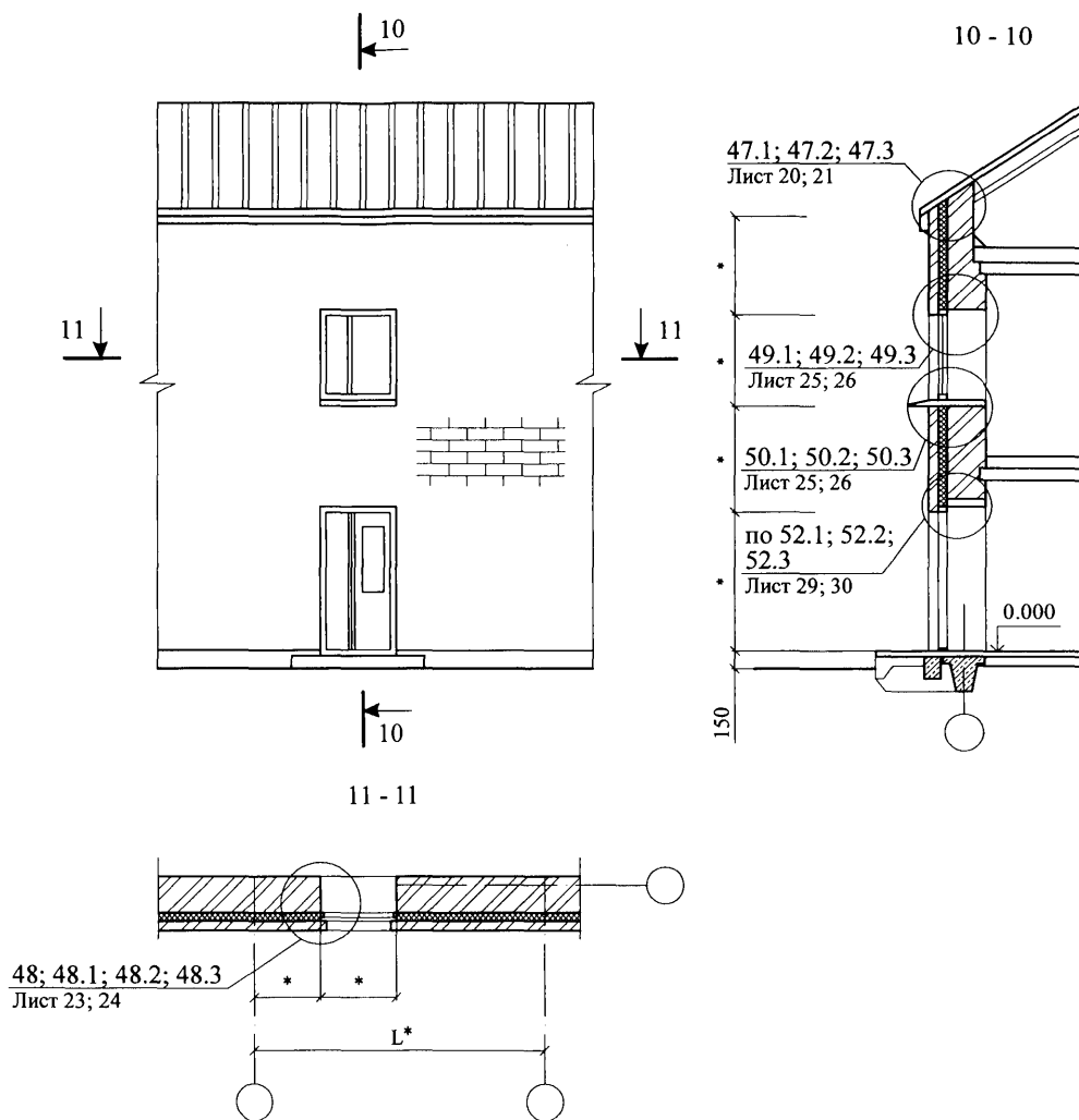
СХЕМА № 9
