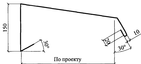
СЛИВ С5
