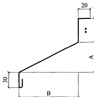
СЛИВ С5
