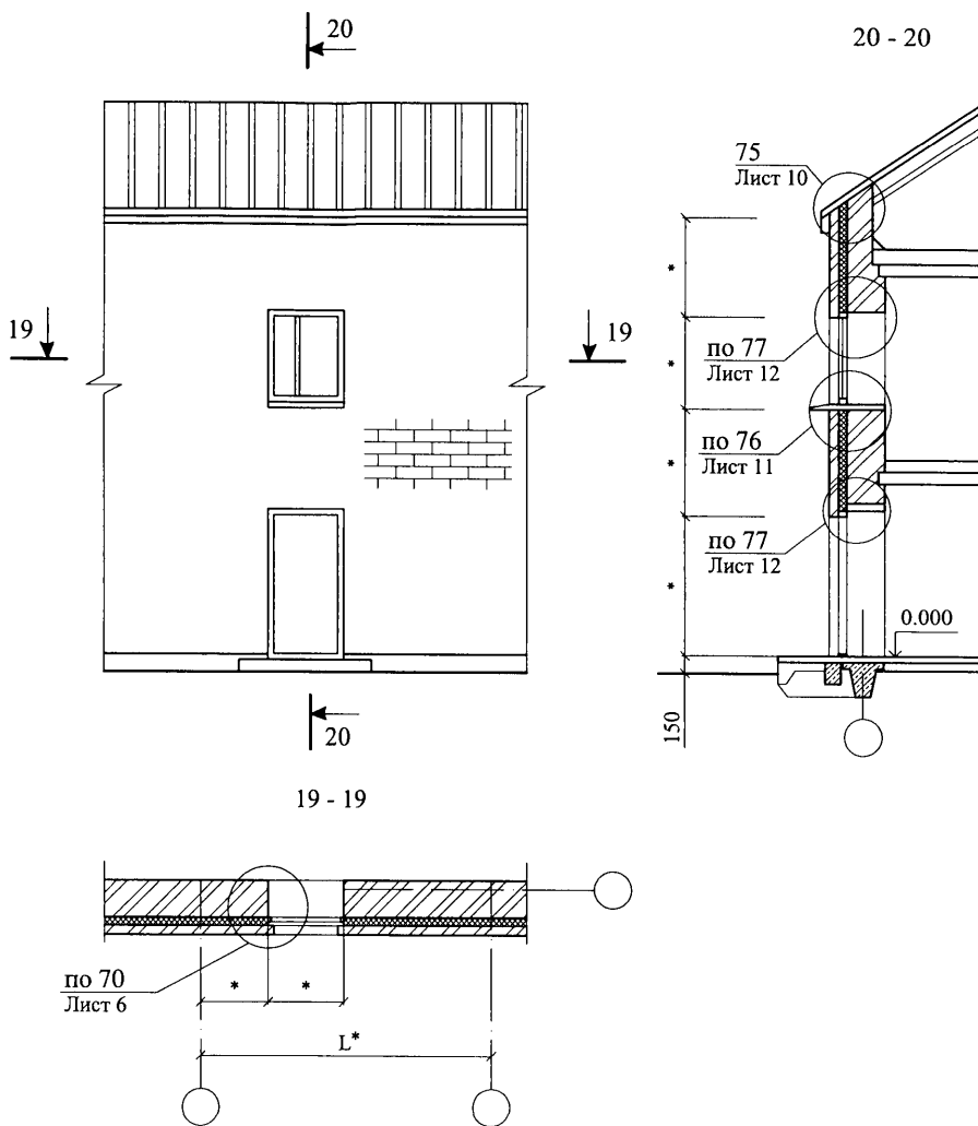
СХЕМА № 15
