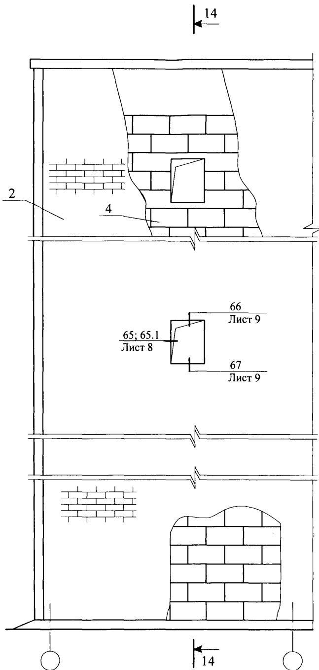
СХЕМА № 11. Расположение плит утеплителя и защитно-декоративной кладки
