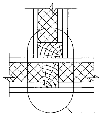
В 1,2 Лист 14
