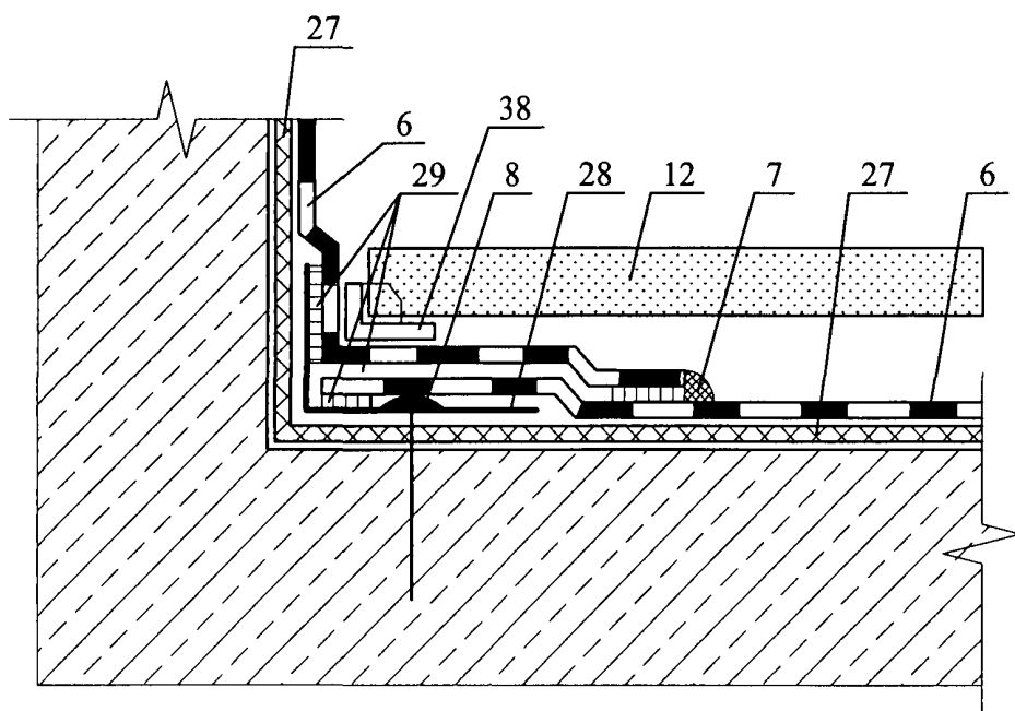
Узел 2.2 - 1
