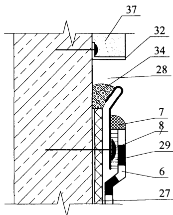
Узел 2.1 - 3
