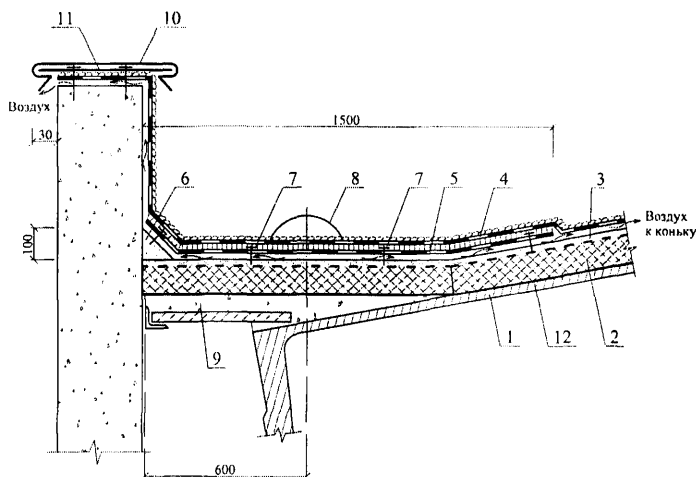
Рис. 11. Примыкание водоизоляционного слоя к парапету
