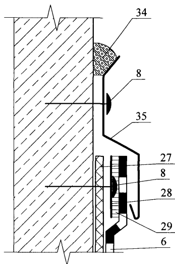
Узел 2.1 - 3
