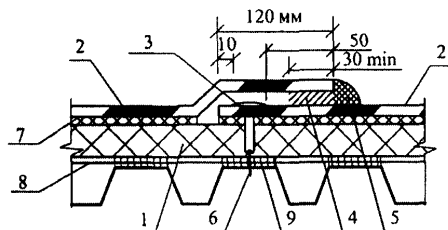
Рис. 18. Стык смежных полотен рулонного материала
