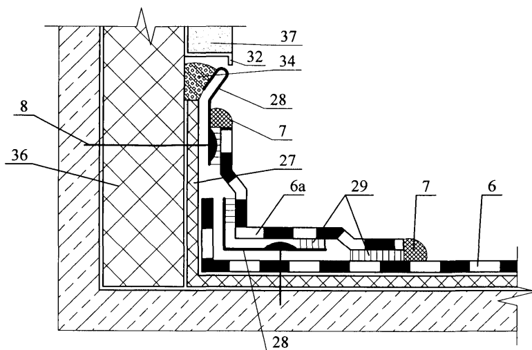
Узел 1.2 - 5
