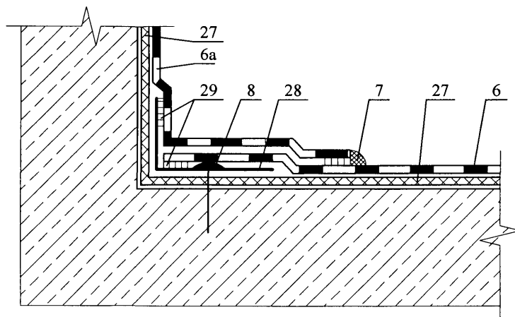
Узел 1.2 - 1
