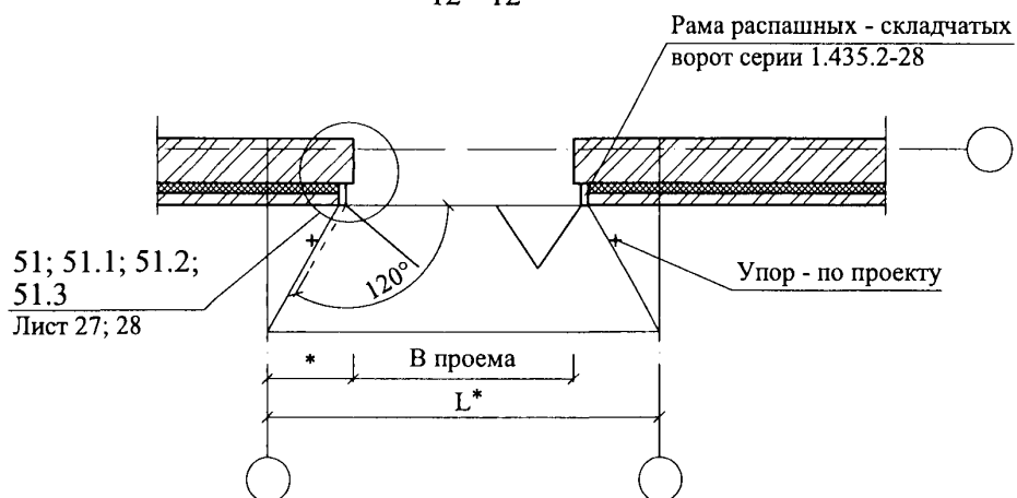
12 - 12
