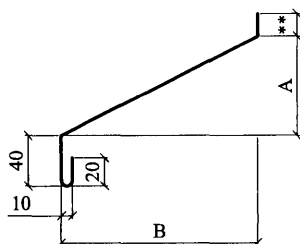
СЛИВ С1
