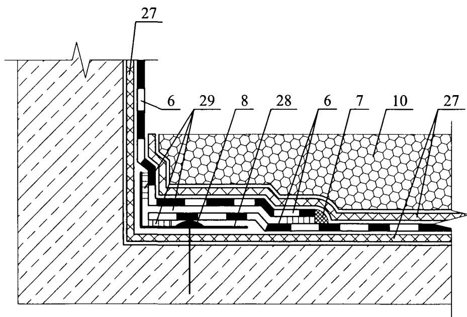
Узел 2.2 - 2
