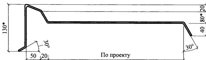
КОСТЫЛЬ К3
