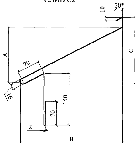
СЛИВ С2
