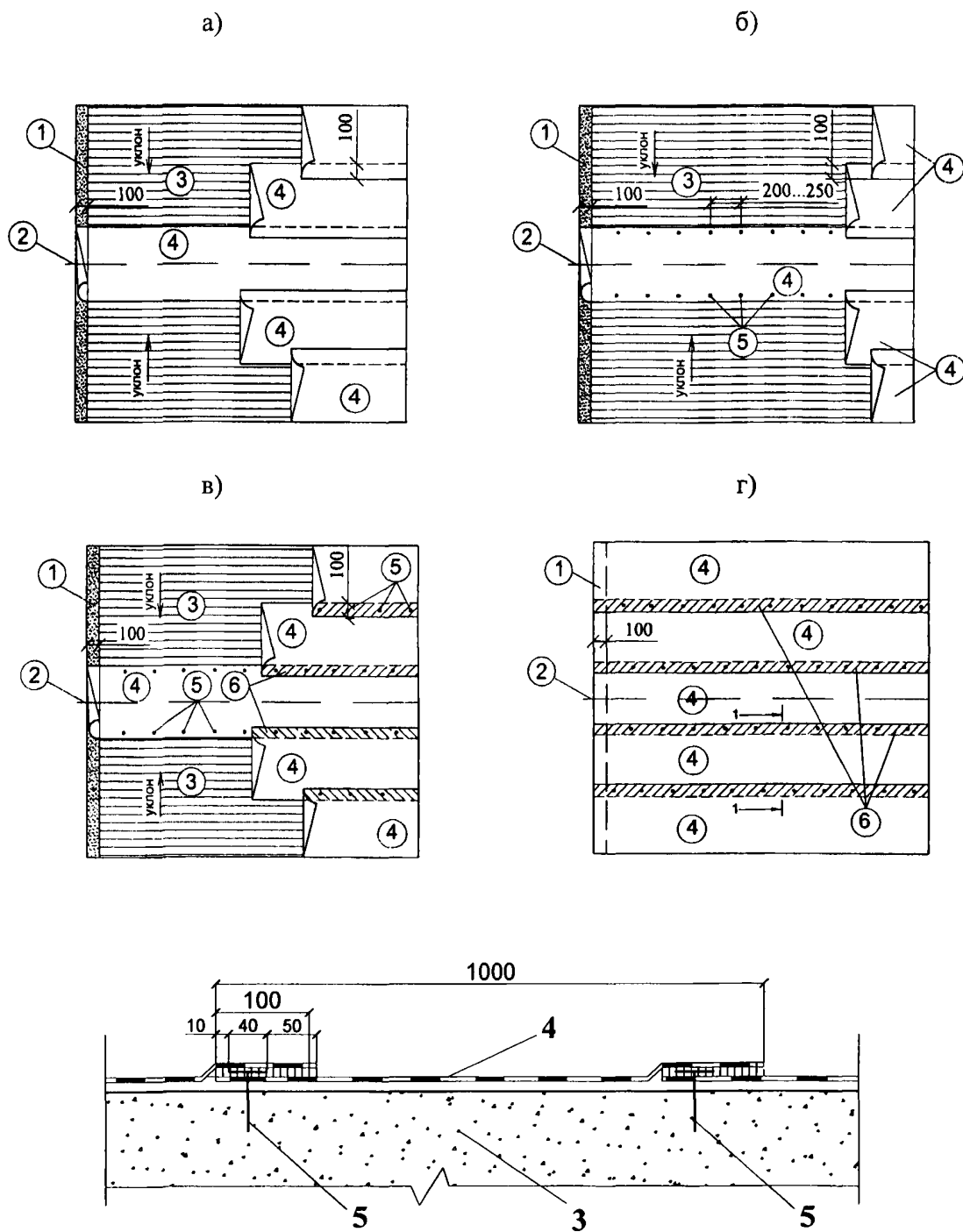
Рис. 2. Раскладка нижнего слоя водоизоляционного ковра из рулонного битумно-полимерного материала с механическим закреплением
