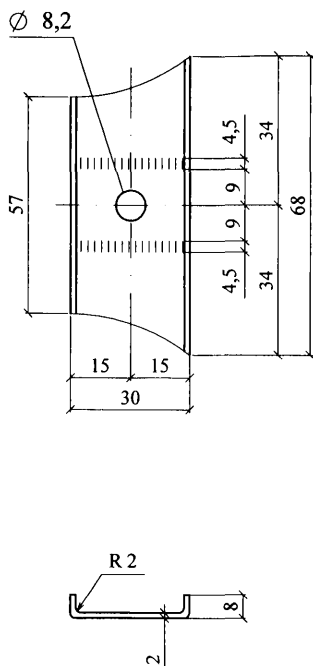
ШАЙБА
