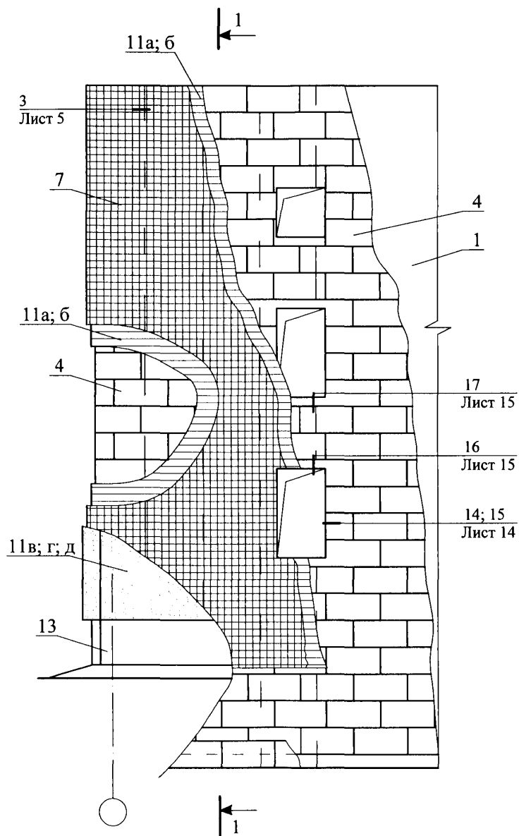
СХЕМА № 1. Расположение плит утеплителя, сетки и штукатурки
