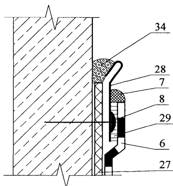
Узел 2.1 - 2
