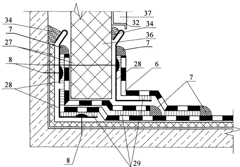
Узел 1.2 - 6
