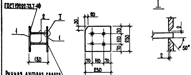
Ручная дуговая сварка в раззенкованных отверстиях электродов типа Э42А
