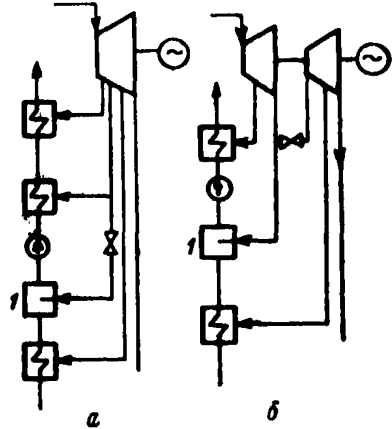
Включение деаэратора в тепловую схему турбоагрегата
