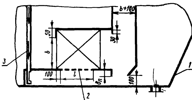
1 — бак-аккумулятор; 2 — барботажный лист; 3 — подвод пара на барботаж; b — высота барботажного канала; l — длина перфорированной части барботажного листа; h_p — высота перегородки
