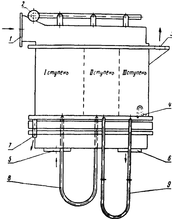
Обвязка эжектора ЭП-3-25/75
