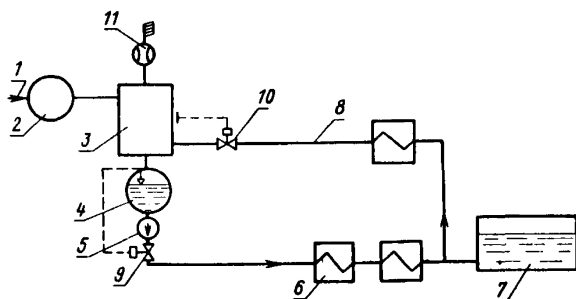
Схема деаэрации подпиточной воды при температуре 45\text{—}50^{\circ}\text{C} с последующим подогревом до 70^{\circ}\text{C}
