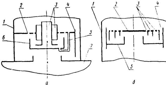
Барботажные устройства деаэраторов повышенного давления конструкции ЦКТИ — БКЗ
