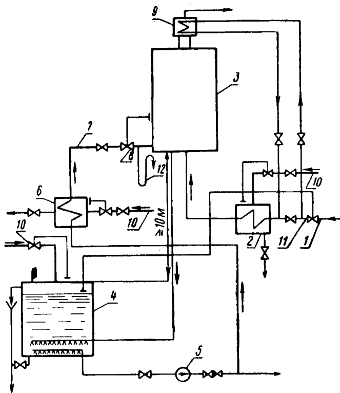
Схема включения вакуумных деаэраторов без потери конденсата
