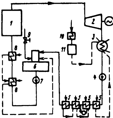
Одноступенчатая схема деаэрации воды
