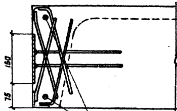
Узел Ж
