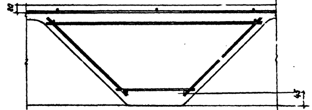
Узел В
