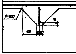
Узел Б
