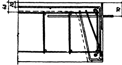
Узел Д
