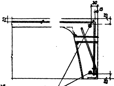
Узел Г
