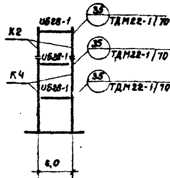
Схема продольной рамы
