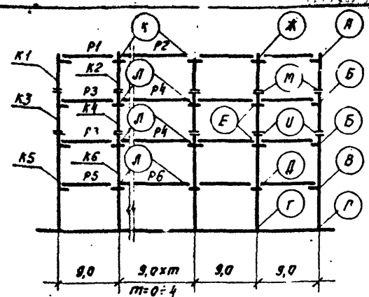
Схема поперечной рамы
