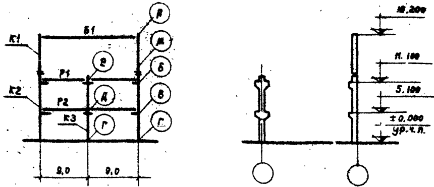
Схема рамы
