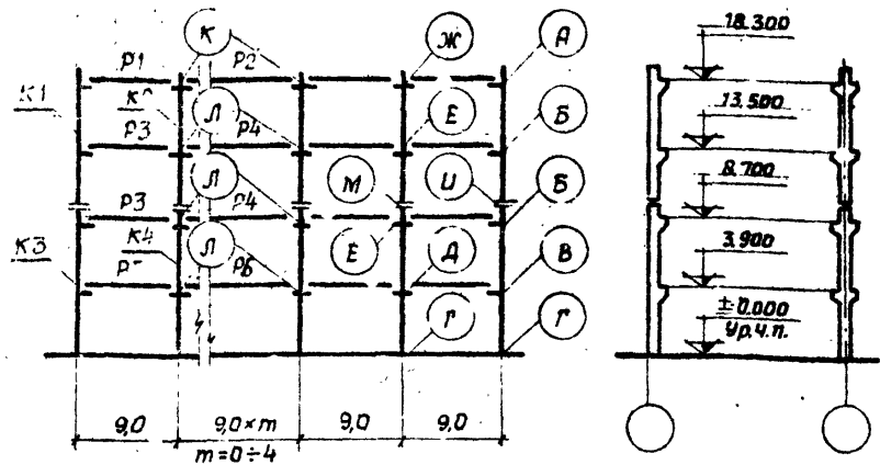
Схема поперечной рамы
