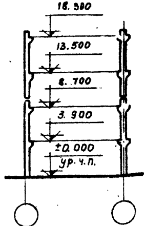
Схема поперечной рамы
