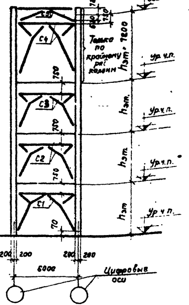
Шифр габаритных схем 2-9-4(48,48,72); 2-9-4(60,60,72)
