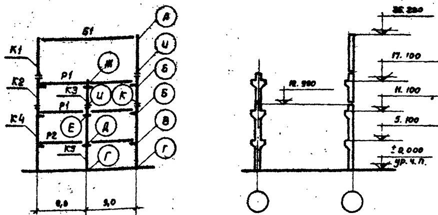
Схема рамы
