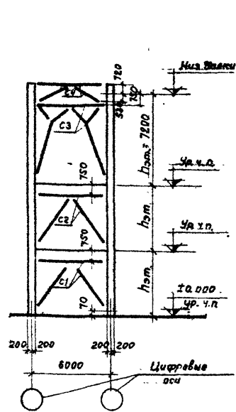
Шифр габаритных схем 2-9-3 (60; 60; 72)
