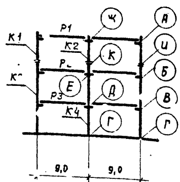
Схема поперечной рамы
