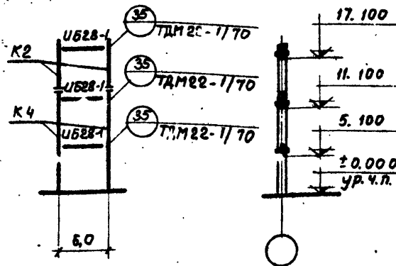
Схема продольной рамы
