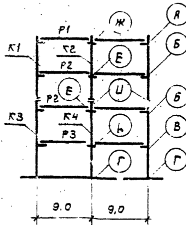
Схема поперечной рамы
