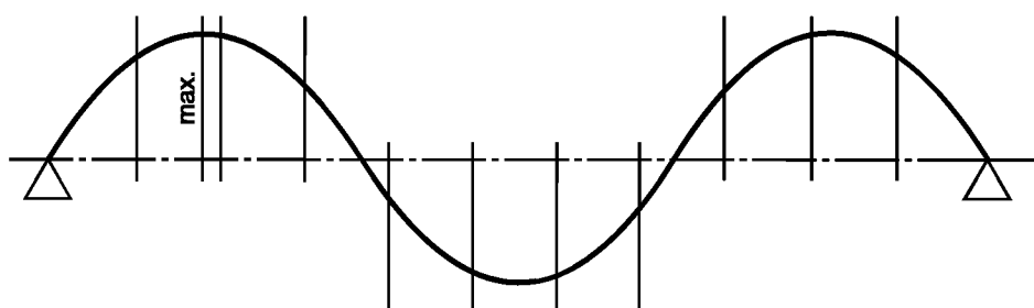
в) Третья мода изгибных колебаний \phi_3(z)
