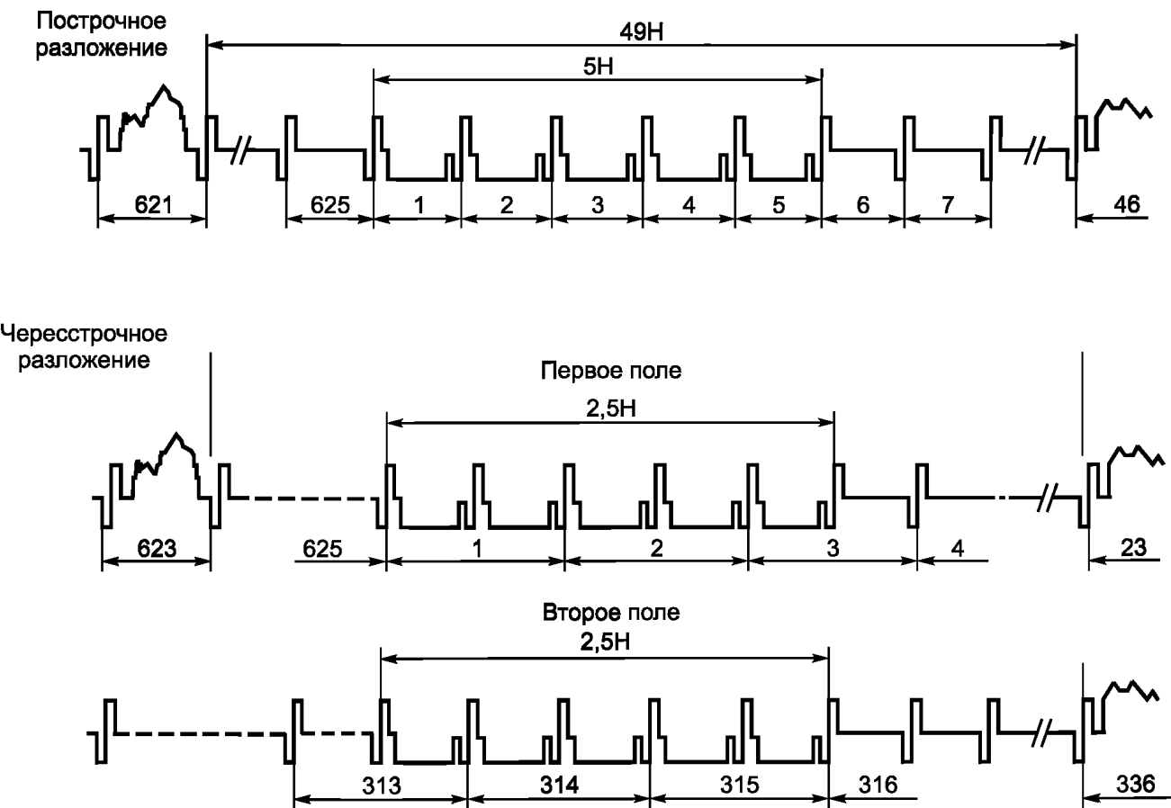
Рисунок 3 — Структура синхросигнала на интервале гашения поля
