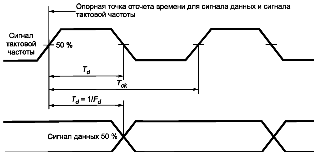
Рисунок 9 — Соотношения параметров синхронизации сигнала и данных
