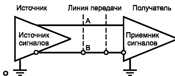
Рисунок 10 — Соединение источника сигналов и приемника сигналов
