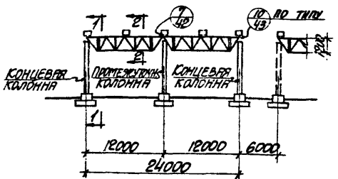
МОНТАЖНАЯ СХЕМА ТЕМПЕРАТУРНОГО БЛОКА L=24.0м ШАГ КОЛОНН 12м. ШАГ ТРАВЕРС 6.0м (ДЛЯ ЭСТАКАД ТИПОВ Iк, IIк)
