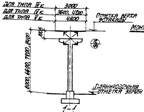
(ДЛЯ ЭСТАКАД ТИПОВ IIIк-IVк)
