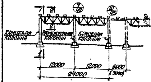
МОНТАЖНАЯ СХЕМА ТЕМПЕРАТУРНОГО БЛОКА L=24.0м. ШАГ КОЛОНН 12м. ШАГ ТРАВЕРС 3.0м (Для эстакад типов Йк; Йк)
