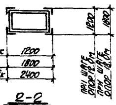
МОНТАЖНЫЕ СХЕМЫ ТЕМПЕРАТУРНЫХ БЛОКОВ L=36.0÷72.0м. ШАГ КОЛОНН 12м. ШАГ ТРАВЕРС 3.0м (Для эстакад типов Йк; Йк)
