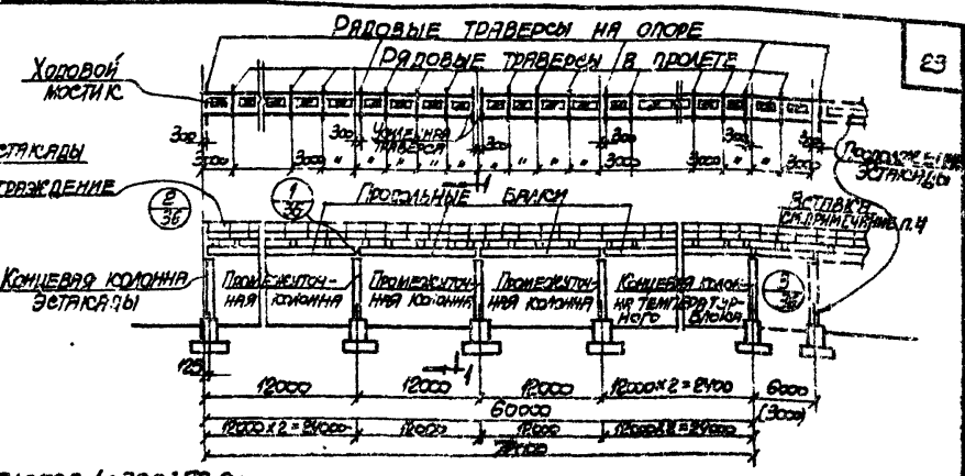
Монтажные схемы температурных блоков L=36,0÷72,0 м
