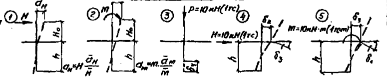
Рис. Расчетные схемы
