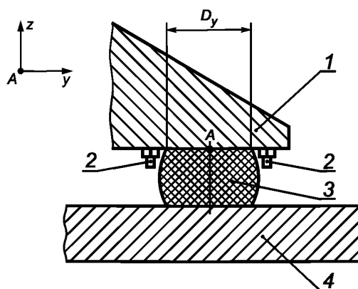
Рисунок 5 — Установка двух акселерометров для измерений v_z
