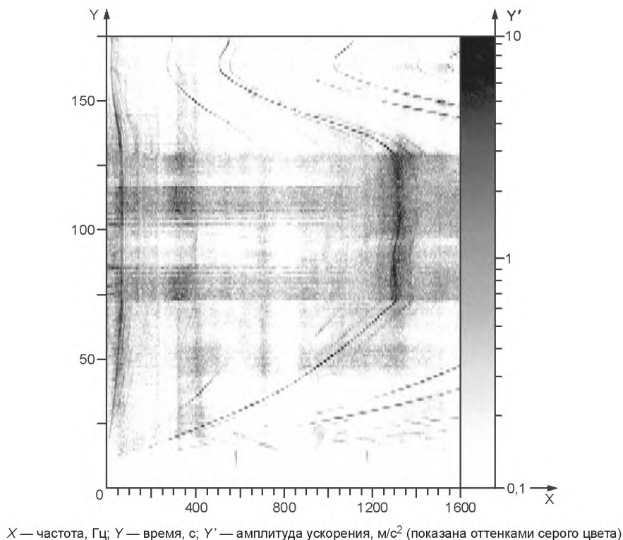
Рисунок 25 — Двумерная спектрограмма
