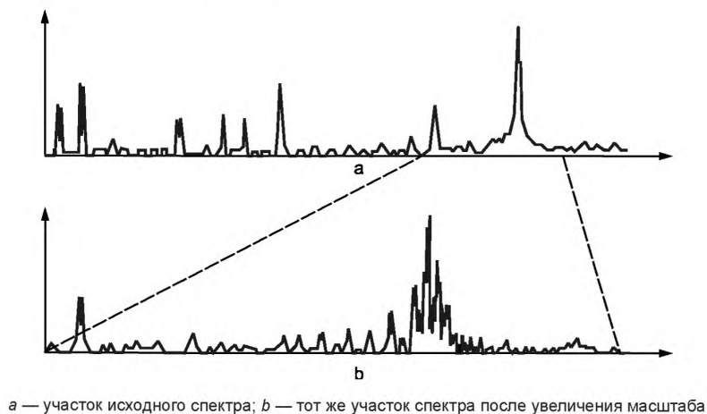
Рисунок 20 — Увеличение масштаба
