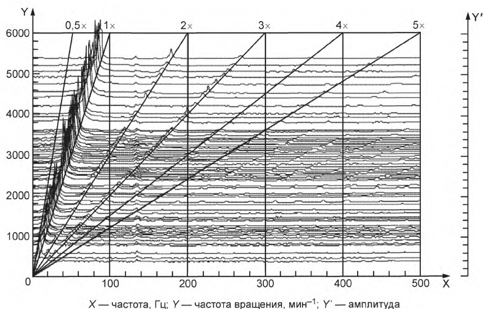
Рисунок 23 — Каскадный спектр
