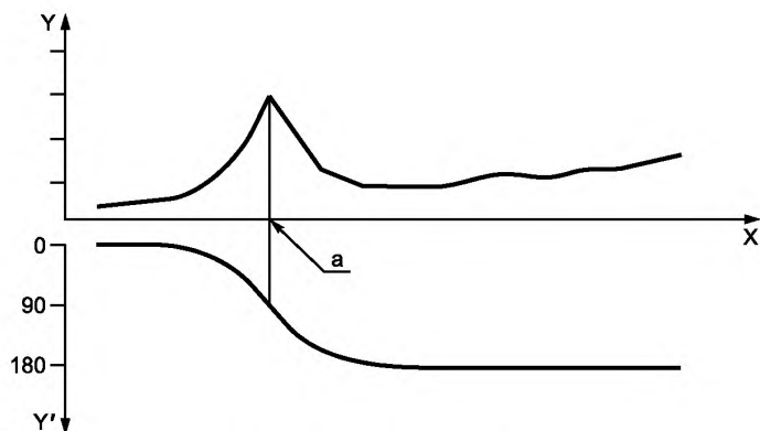
Рисунок 21 — Диаграмма Бode
