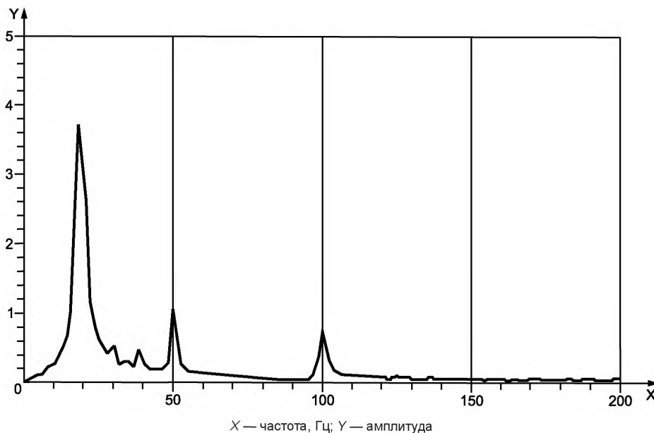
Рисунок 16 — Амплитудный спектр
