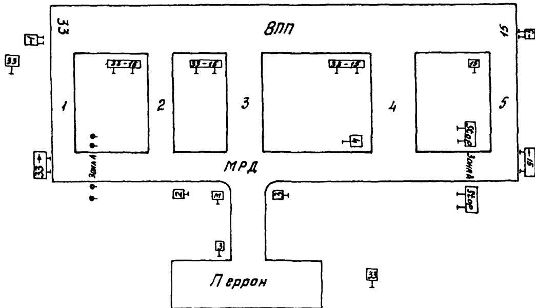
Рис. II. Размещение неуправляемых световых указателей: 33 - неуправляемый световой указатель
