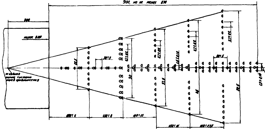
Рис. 4. Схема расположения огней приближения и световых горизонтов системы точного захода на посадку по категории I (ОВИ-I): □ - огни приближения и световых горизонтов прожекторные белые; ○ - огни приближения и световых горизонтов кругового обзора белые.
