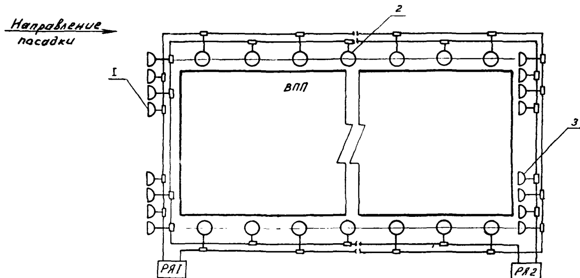
Рис. 22. Схема электропитания посадочных огней линзового типа, входных и ограничительных огней прожекторного типа систем ОВИ-1: 1 - прожекторный огонь входной; 2 - линзовый огонь ВПП высокой интенсивности; 3 - прожекторный огонь ограничительный
