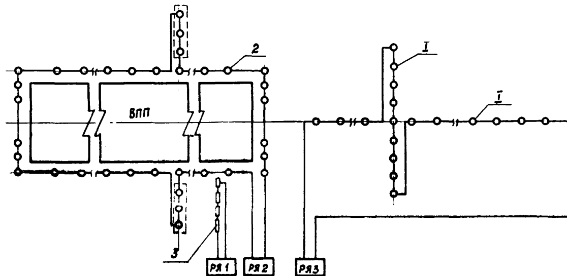
Рис. 24. Схемы электропитания огней в светосигнальных системах ОМИ: I - огни приближения и светового горизонта кругового обзора; 2 - огни ВПП; 3 - галесадные огни
