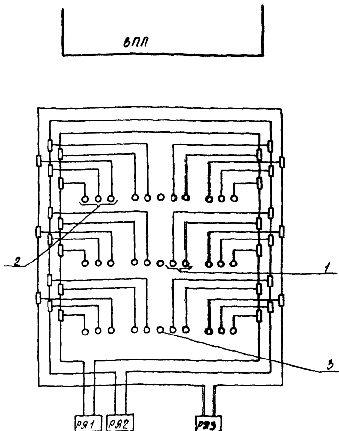
Рис. 13. Схема электропитания прожекторных огней центрального ряда и боковых огней на КЛБ систем ОБИ-2 со световыми горизонтами: 1 - огни КЛБ центрального ряда прожекторные; 2 - огни КЛБ бокового ряда прожекторные; 3 - осевые огни КЛБ прожекторные
