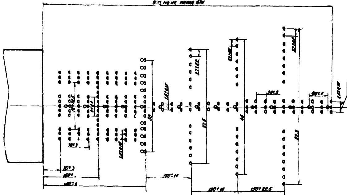
Рис. 7. Схема расположения огней приближения систем точного захода на посадку по категории II (ОВУ-2): ● - боковые огни КЛБ прожекторные красные; □ - огни приближения и светового горизонта прожекторные белые; ○ - огни приближения и светового горизонта кругового обзора белые.
