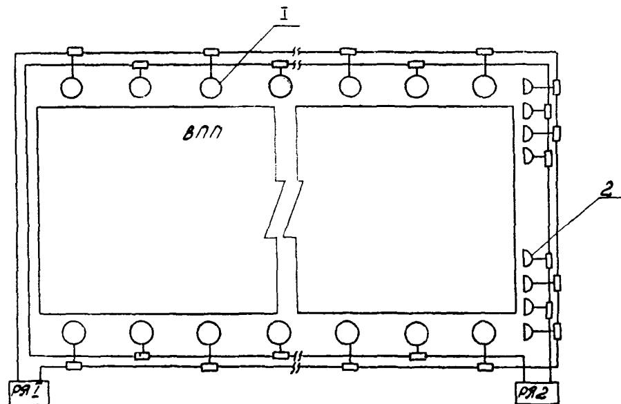
Рис. 23. Схема электропитания посадочных огней линзового типа и ограничительных огней прожекторного типа систем ОВИ-2 и ОВИ-3: 1 - линзовый огонь ВПТ высокой интенсивности; 2 - прожекторный огонь ограничительный
