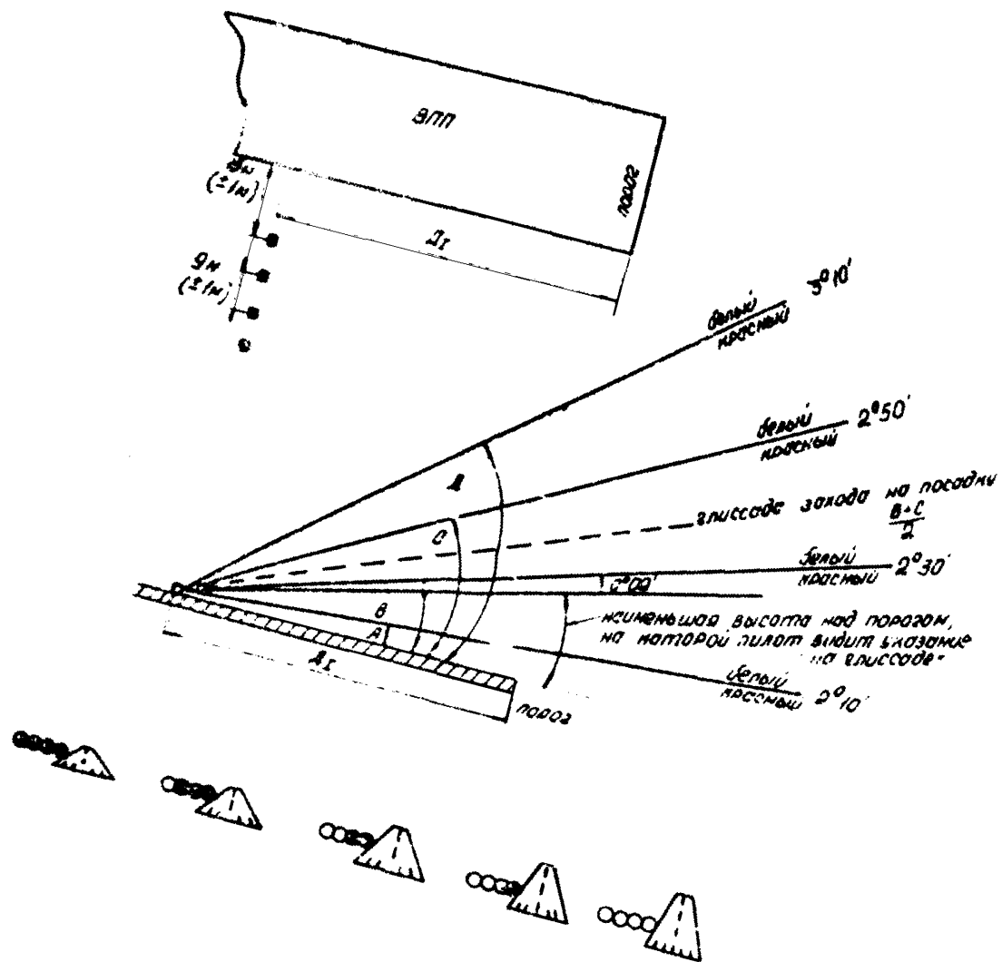
Схема расположения огневой системы ПАРУ и распределе- ние углов захода на посадку (угол захода на посадку 20°40')
