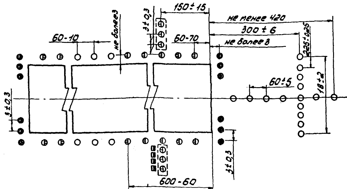
Рис. 1. Схема расположения светосигнального оборудования системы ОМИ для полетов по ПВП: ○ - огонь приближения и светового горизонта; ● - входной ограничительный огонь зеленый-красный; ⊕ - посадочный огонь ВПП белый-желтый; ⊕ - огонь знака приземления белый; □ - глиссадный огонь
