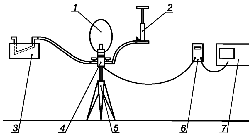
1 — надувная оболочка; 2 — воздушный насос; 3 — манометр; 4 — приспособление с микрофоном; 5 — тренога; 6 — частотный модулятор; 7 — осциллограф
