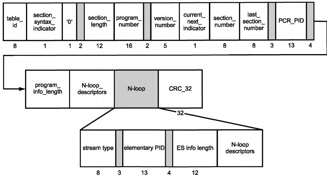
Рисунок А.5 — Структура полей секции таблицы PMT
