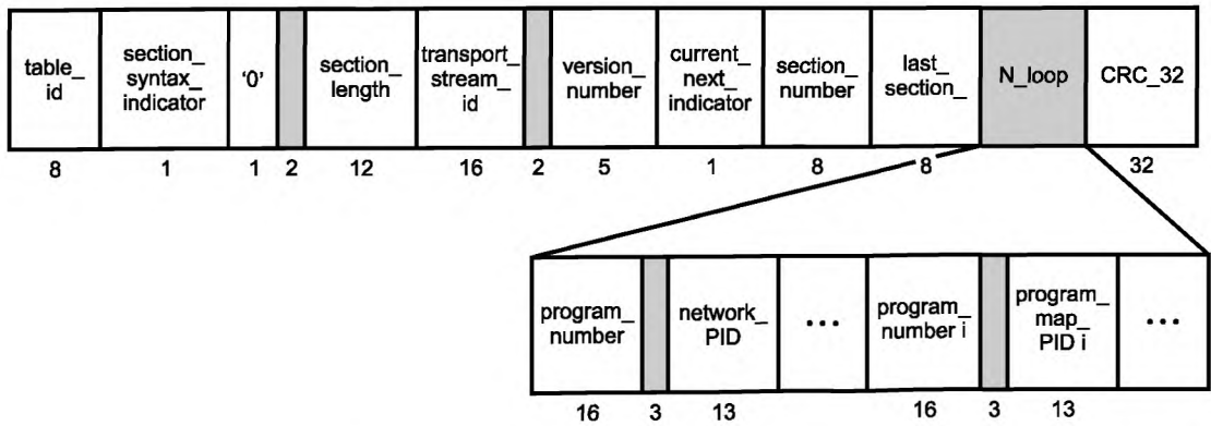
Рисунок А.3 — Структура полей секции таблицы PAT
