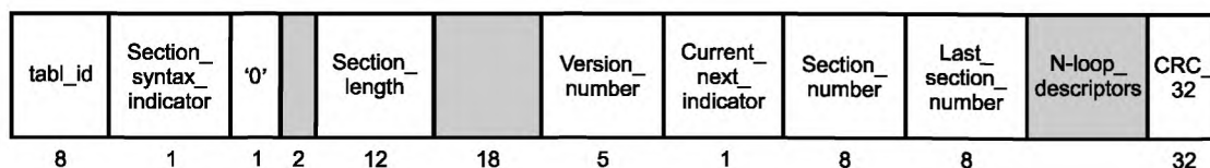
Рисунок A.4 — Структура полей секции таблицы CAT
