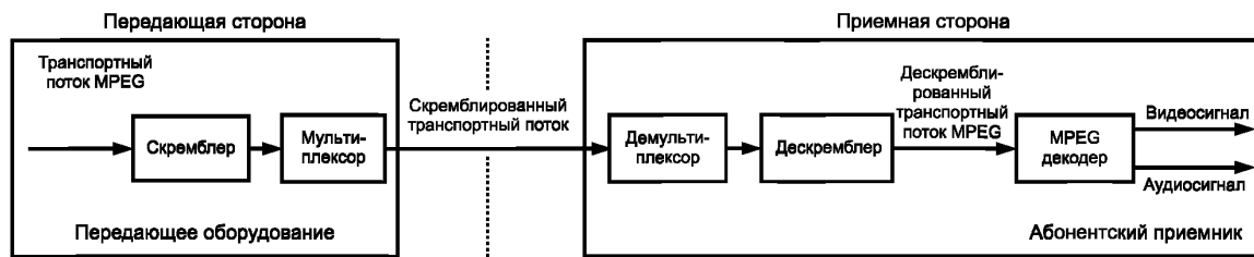
Рисунок 1 — Структурная схема одноуровневой СОД
