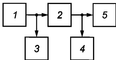
Рисунок 4 — Схема измерения коэффициента нелинейных искажений
