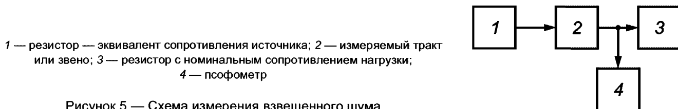
Рисунок 5 — Схема измерения взвешенного шума
