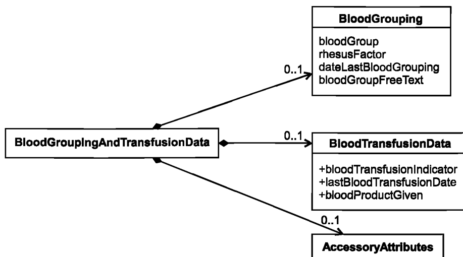
Рисунок 5 — Структура класса информационных объектов «BloodGroupingAndTransfusionData»
