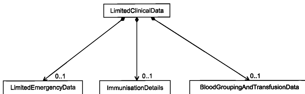
Рисунок 2 — Структура класса «LimitedClinicalData»
