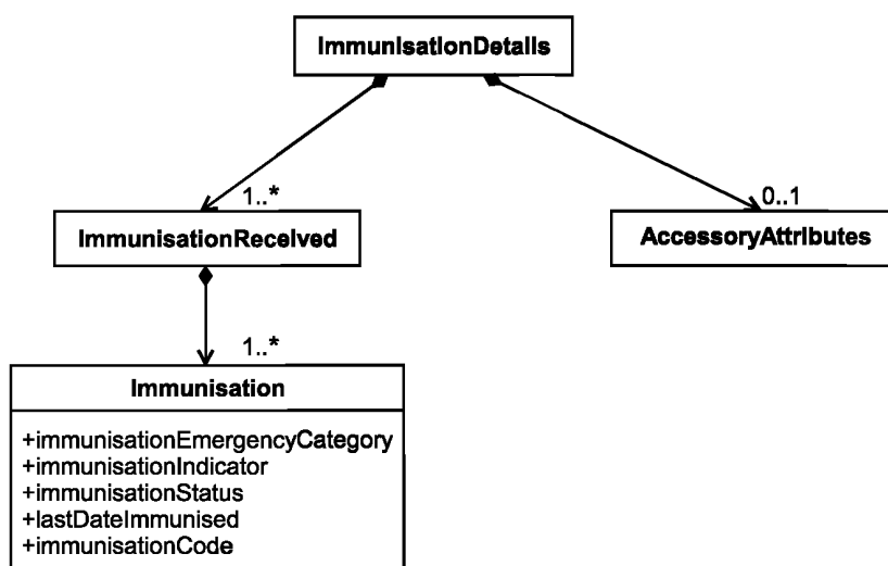
Рисунок 4 — Структура класса информационных объектов «ImmunizationDetails»
