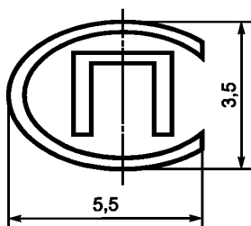
Рисунок А.1 — Сталь с пределом пропорциональности \sigma_g \geq 450 МПа
