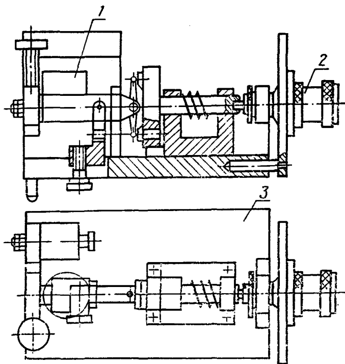
1—индикатор; 2—микрометрическая головка; 3—плита
