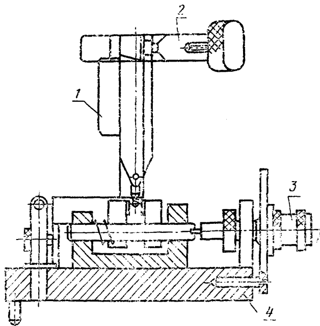
1—индикатор; 2—зажимы; 3—микрометрическая головка; 4—плита
