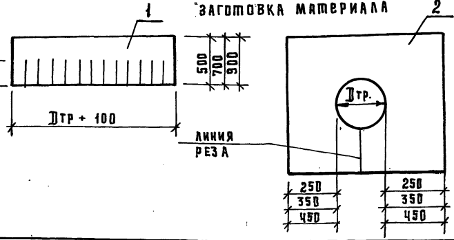
ЗАГОТОВКА МАТЕРИАЛА
