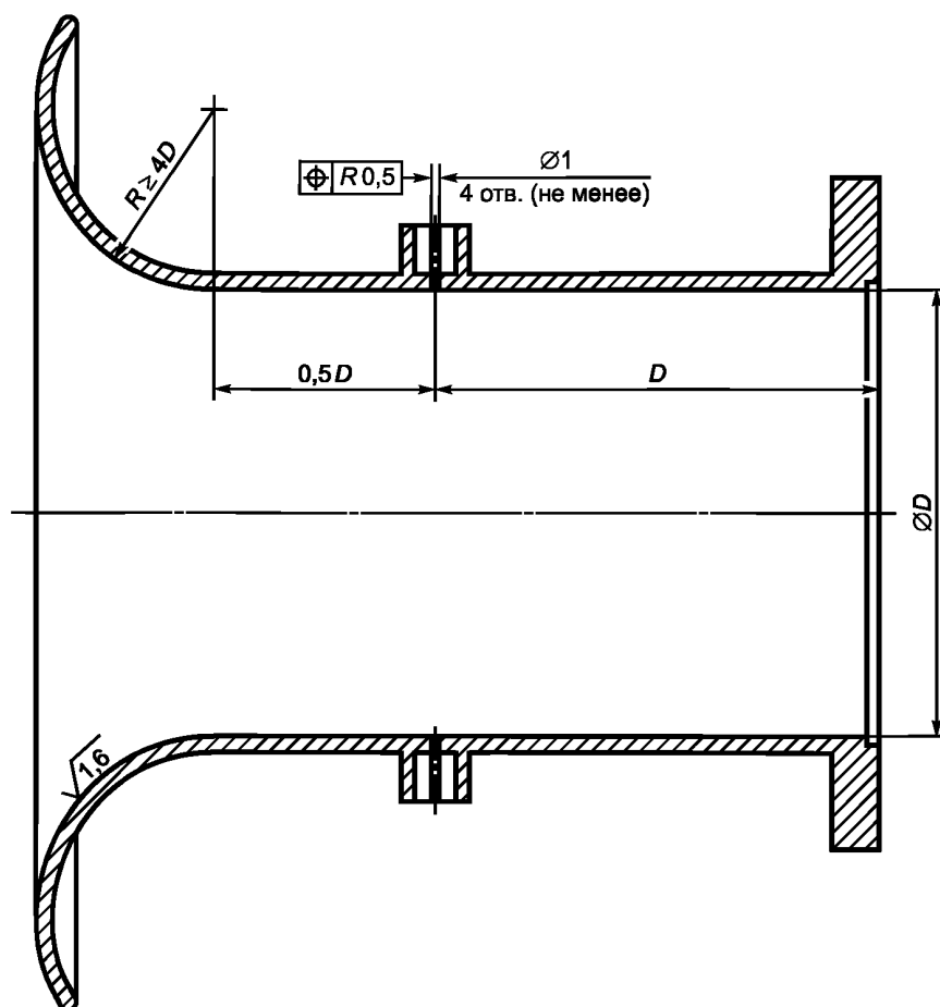
Рисунок 1 — Коллектор для измерения расхода воздуха
