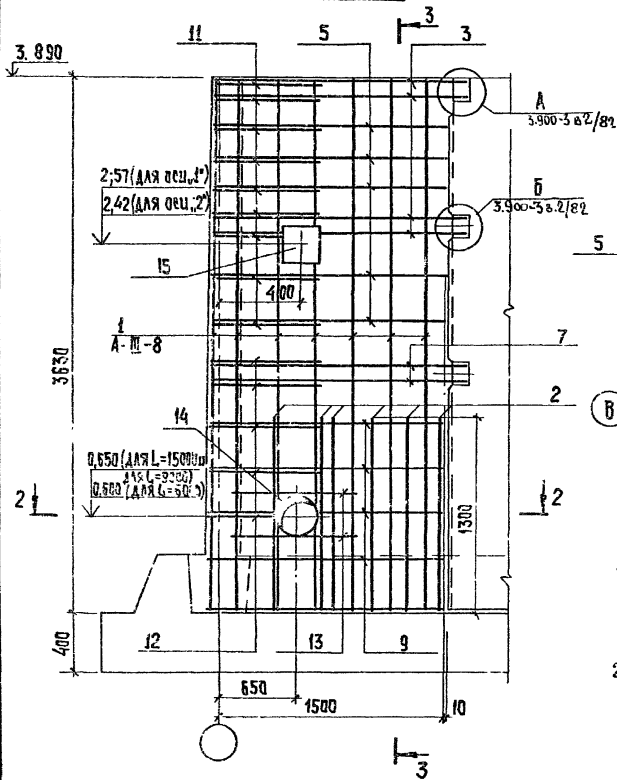
РАЗРЕЗ 1-1
