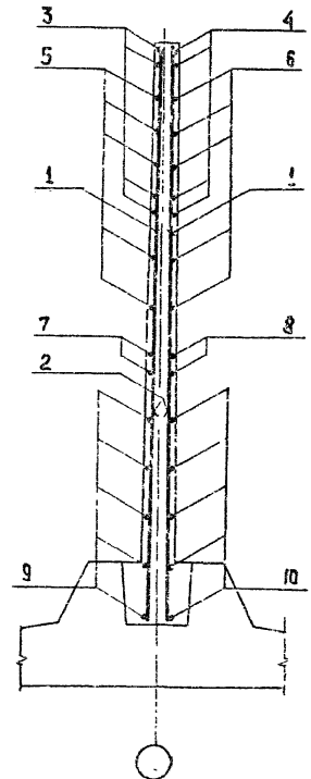
РАЗРЕЗ 3-3
