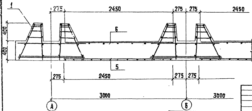
РАЗРЕЗ 1-1
