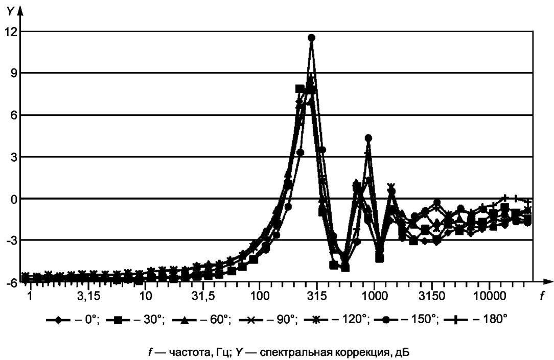
Рисунок С.2 — Спектральная коррекция на влияние отражений от земли в зависимости от направления распространения дутьевой волны
