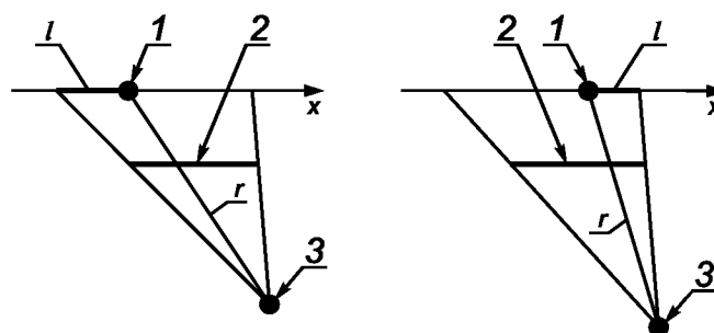
Рисунок А.2 — Экранирующий эффект препятствия
