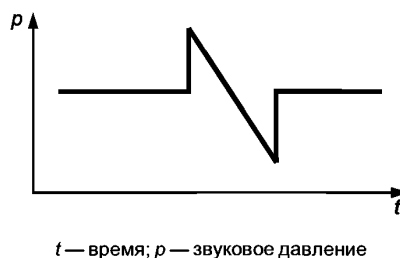
Рисунок 2 — Зависимость от времени звукового давления сверхзвуковой пули в N-волне
