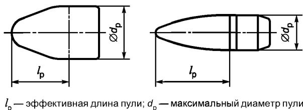
Рисунок 1 — Эффективная длина пули
