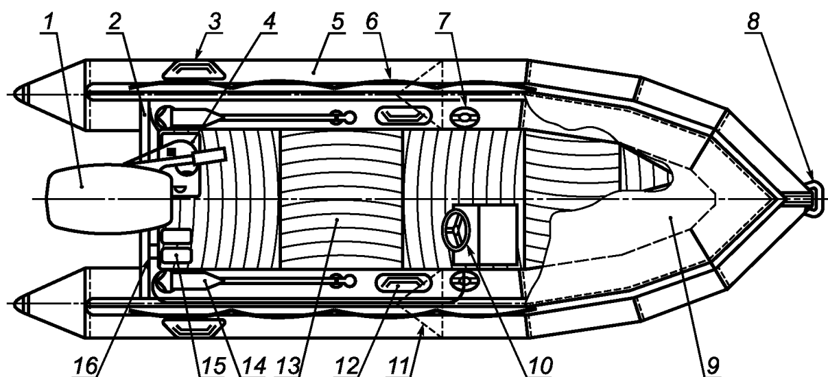
Общий вид стандартной лодки VII типа
