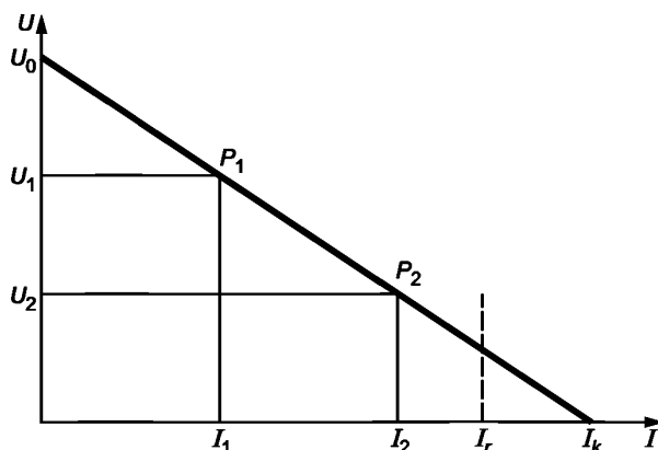
Рисунок 2 — Нагрузочные характеристики генераторов тока
