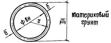
Расчетное сечение
