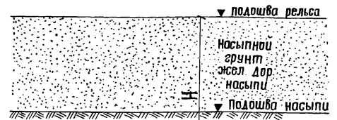
Расчетная схема
