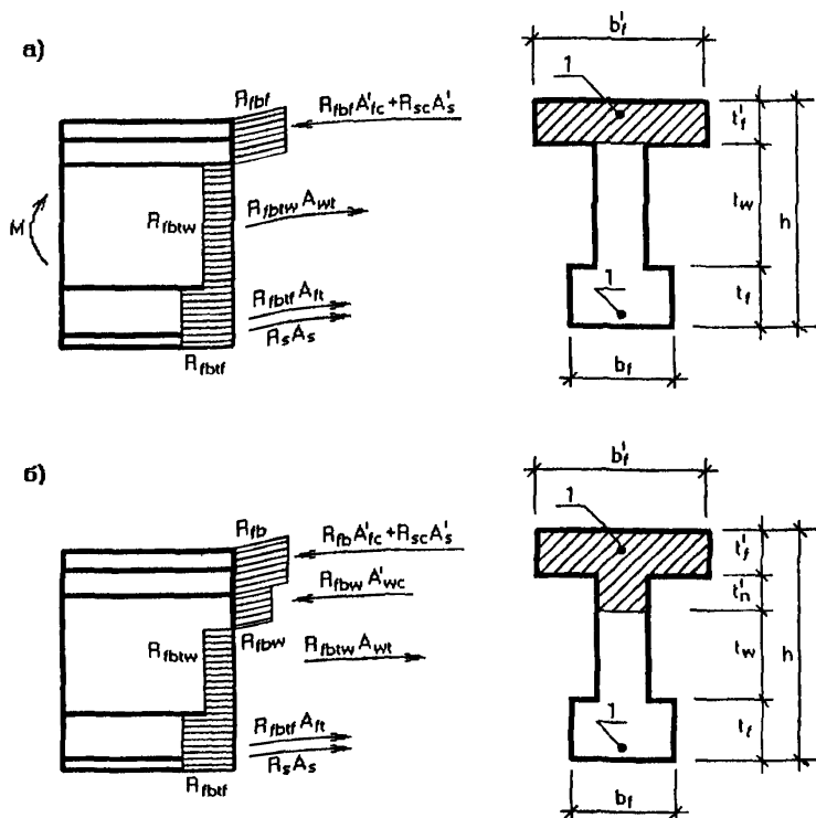
Рис. 4. Схема распределения усилий и эпюра напряжений в сечениях, нормальных к продольной оси изгибаемого элемента двутаврового сечения при комбинированном армировании а – при x \leq x_r' ; б – при x > x_r' ; 1 – стержневая или проволочная арматура.
