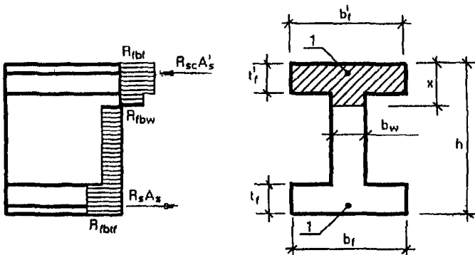
Рис. 1. Схема внутренних усилий и эпюры напряжений в сечении, нормальном к продольной оси элемента (общий случай) 1 – сосредоточенная стержневая или проволоочная арматура
