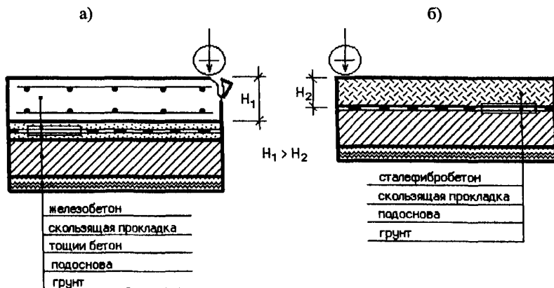
Рис. 1.Ж. Сопоставительные конструктивные решения индустриальных полов по грунтам: а) традиционный железобетонный пол; б) сталефибробетонный пол.
