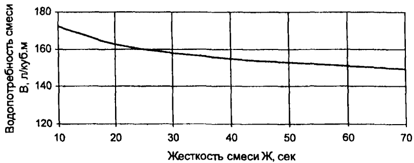
Рис.3. График водопотребности пластичной (а) и жесткой (б) бетонной смеси
