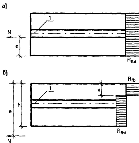
Рис. 7. Эпюры напряжений во внецентренно растянутых элементах прямоугольного сечения а – при приложении продольной силы N в пределах ядра сечения; б – то же, за пределами; 1 – стержневая или проволочная арматура.
