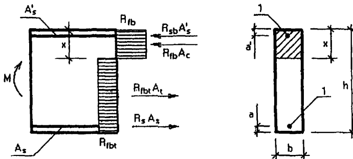
Рис. 3. Схема усилий и эпюра напряжений в сечениях, нормальных к продольной оси изгибаемого железобетонного элемента прямоугольного сечения при комбинированном армировании 1 – стержневая или проволоочная арматура
