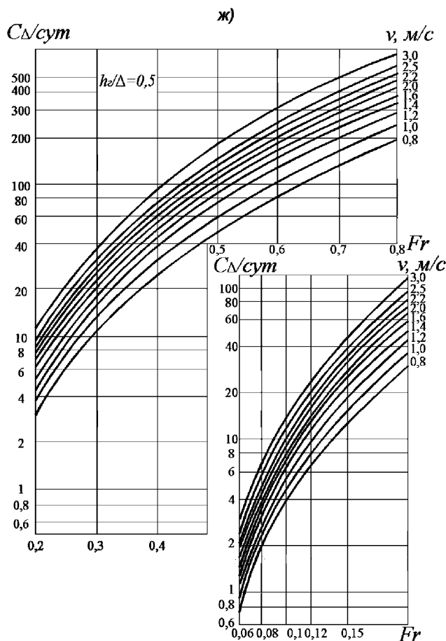
Рисунок 9.4 — Номограммы для определения скорости движения русловых мезоформ с учетом различных значений относительных высот микроформ h_r/\Delta :
