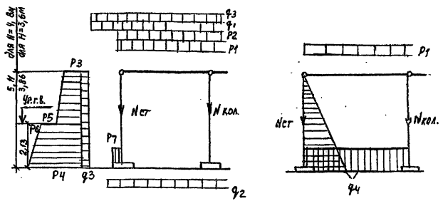
Рис.1 Схемы основных сочетаний нагрузок
