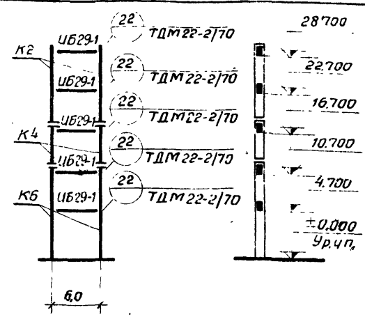
Схема продольной рамы
