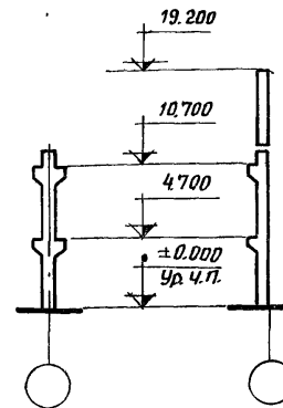
Схема рамы
