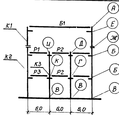
Схема рамы
