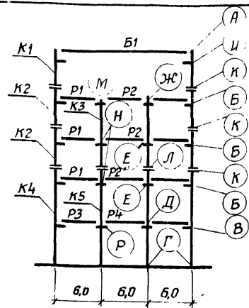
Схема рамы
