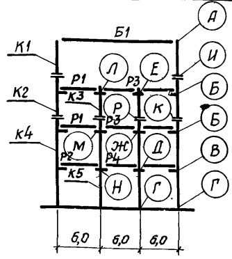
Схема рамы
