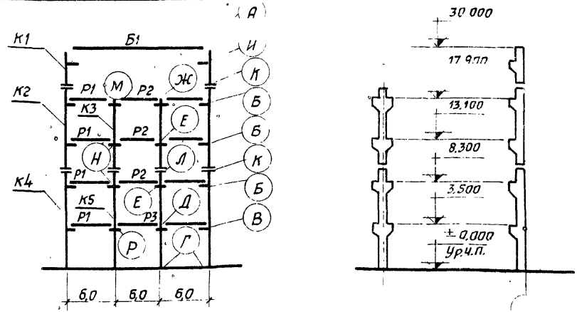
Схема рамы
