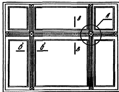
Схемы витрин с уширенными вертикальными и горизонтальными импостами.
