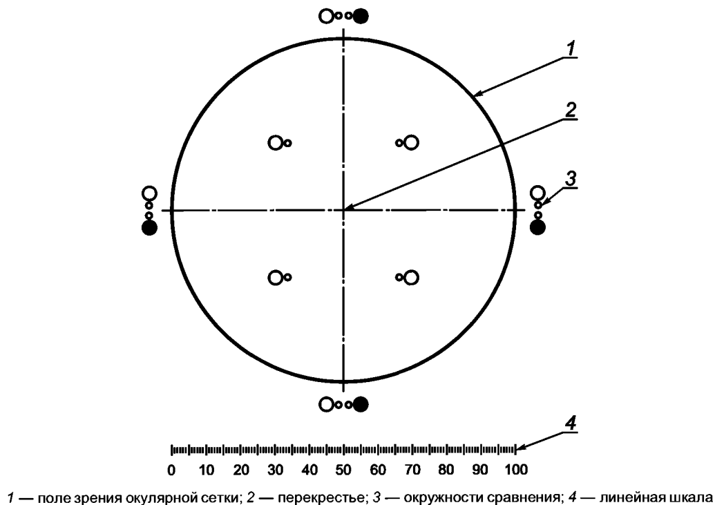
Рисунок Г.1 — Окулярная сетка с окружностями
