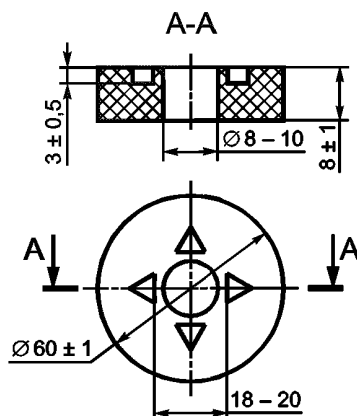
Рисунок А.1 — Подставка для вертикальной печи
