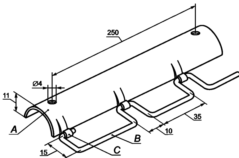
А — стальной желоб диаметром 25 мм и толщиной 1,6 мм; В — поворотные соединения из стальной проволоки диаметром 2,5 мм; С — петли, припаянные к желобу
