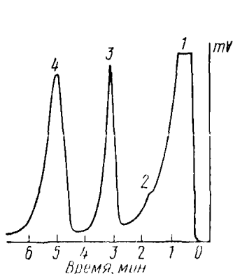
Рис. 4 Хроматограмма экстракта, содержащего дибутилсебацат и дибутилфталат:
