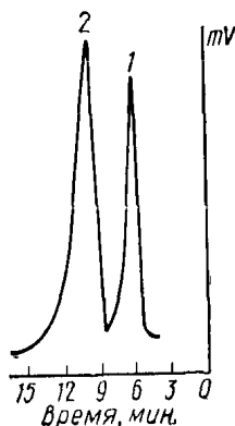
Рис. 5. Хроматограмма экстракта, содержащего диоктилфталат и диамиловый эфир себаценовой кислоты:
