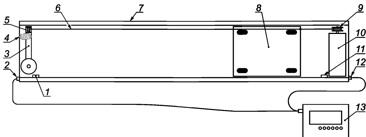
1 — конечный выключатель левый; 2 — разъем подключения кабеля № 2; 3 — рычаг натяжителя; 4 — пружина натяжителя; 5 — ролик натяжителя; 6 — леска привода подвижной тележки; 7 — корпус — направляющая станина; 8 — подвижная тележка; 9 — ролик привода с датчиком импульсов; 10 — мотор привода; 11 — конечный выключатель правый; 12 — разъем подключения кабеля № 1; 13 — пульт управления и индикации
