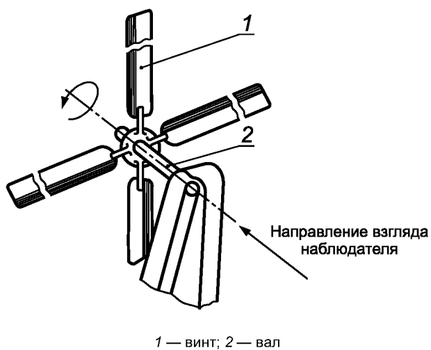
1 — винт; 2 — вал
