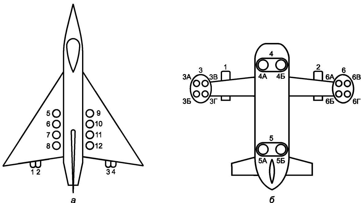
Рисунок 2 — Нумерация подъемных двигателей
