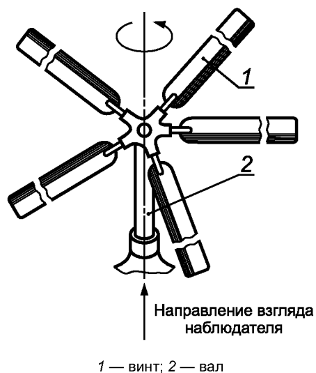
1 — винт; 2 — вал
