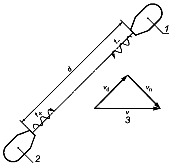
1 — преобразователь–; 2 — преобразователь+; 3 — составляющие скорости ветра
