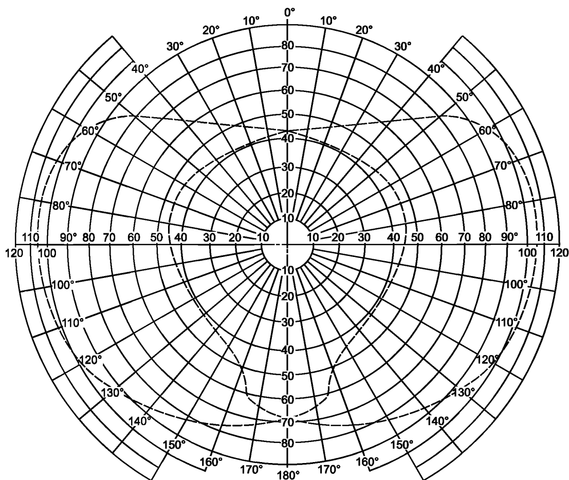
Рисунок 5 — Диаграмма апертометра
