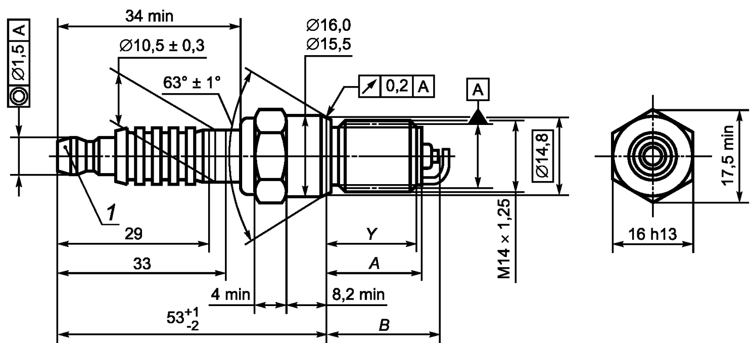
а) со штыревой контактной головкой
