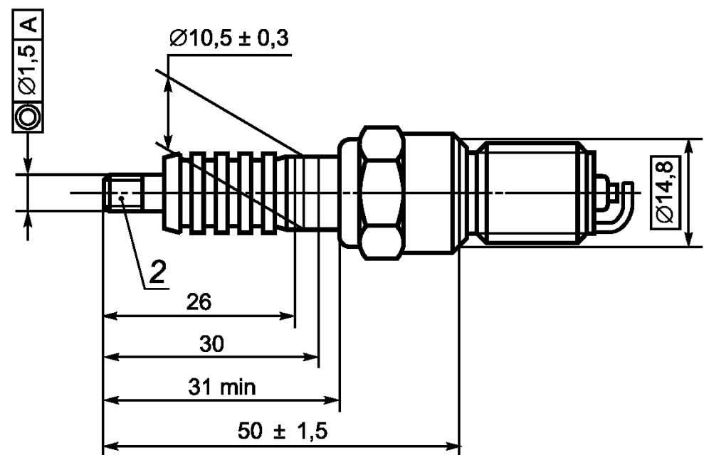
б) с резьбовой контактной головкой
