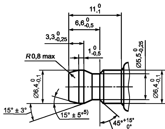
а) штыревая контактная головка
