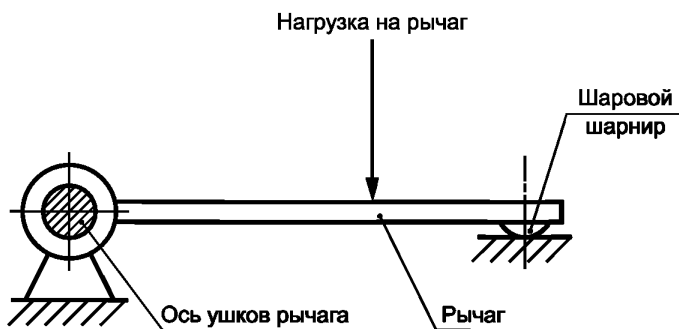
Рисунок 2 — Схема испытаний рычагов на прочность
