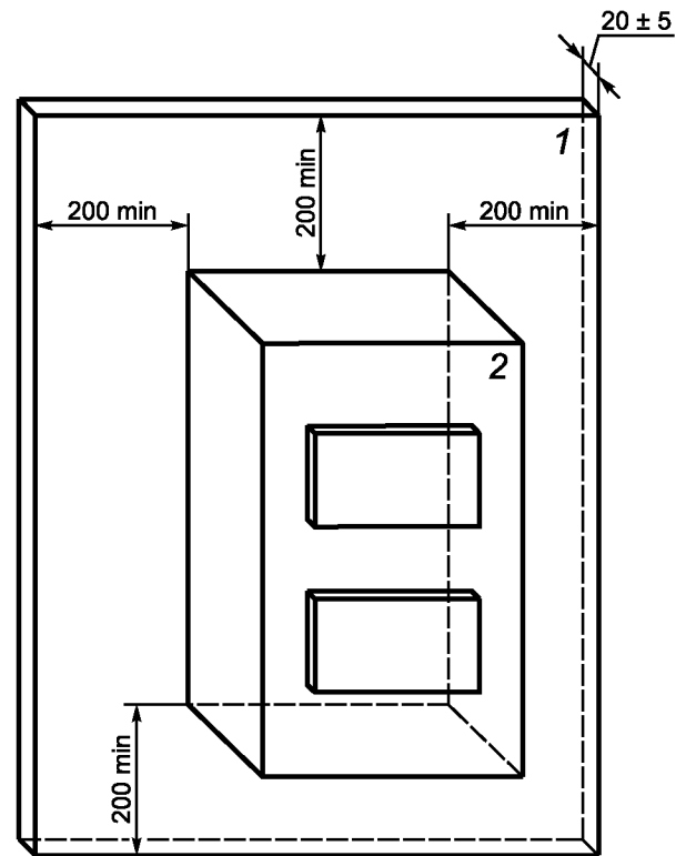
1—фанера; 2 — корпус
