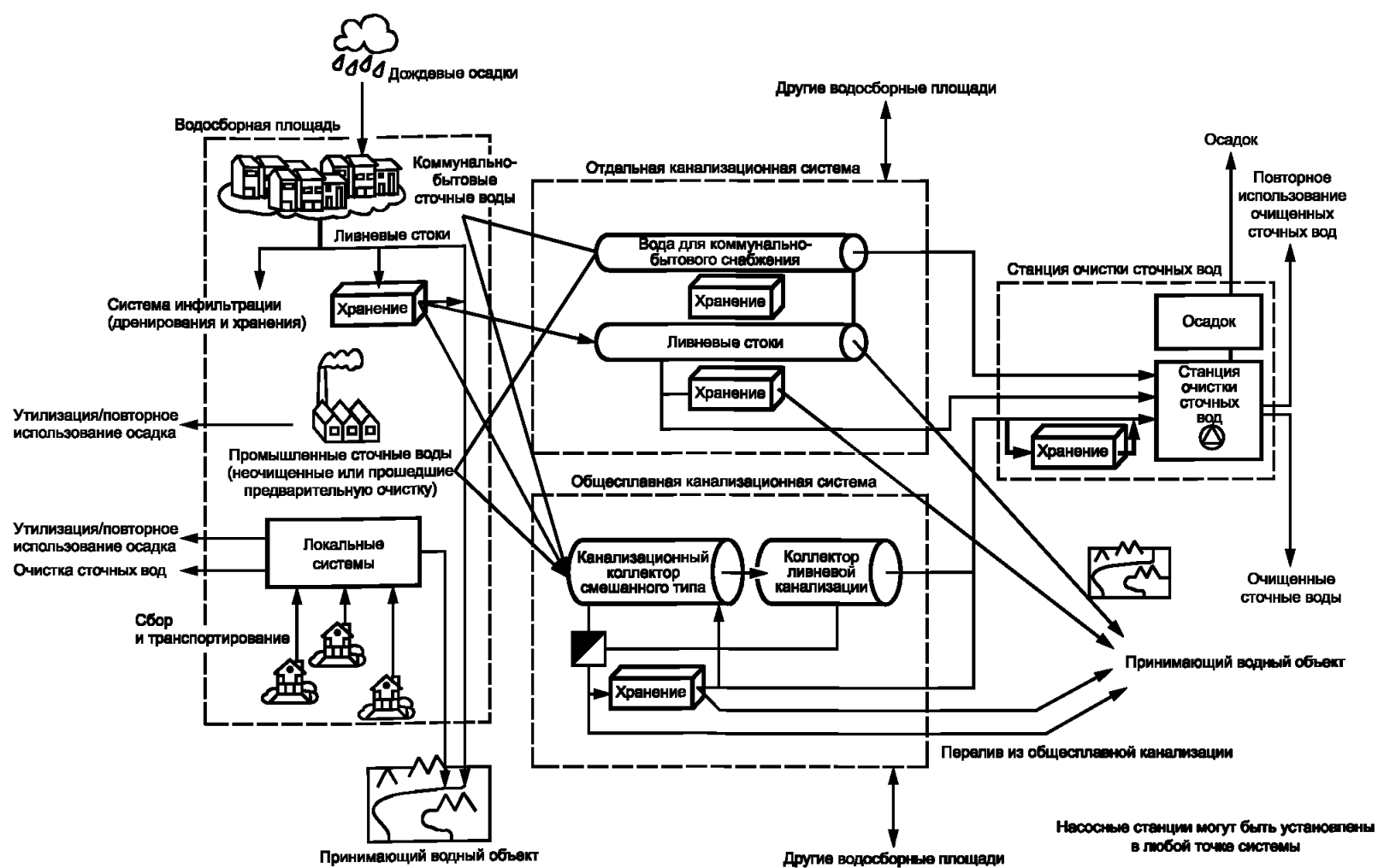
Рисунок В.1 — Схематическое изображение систем удаления сточных вод
