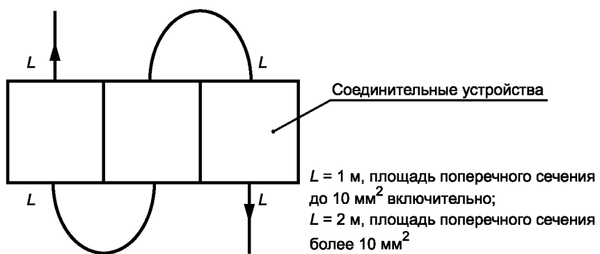
Рисунок 102 — Зажим на несколько направлений
